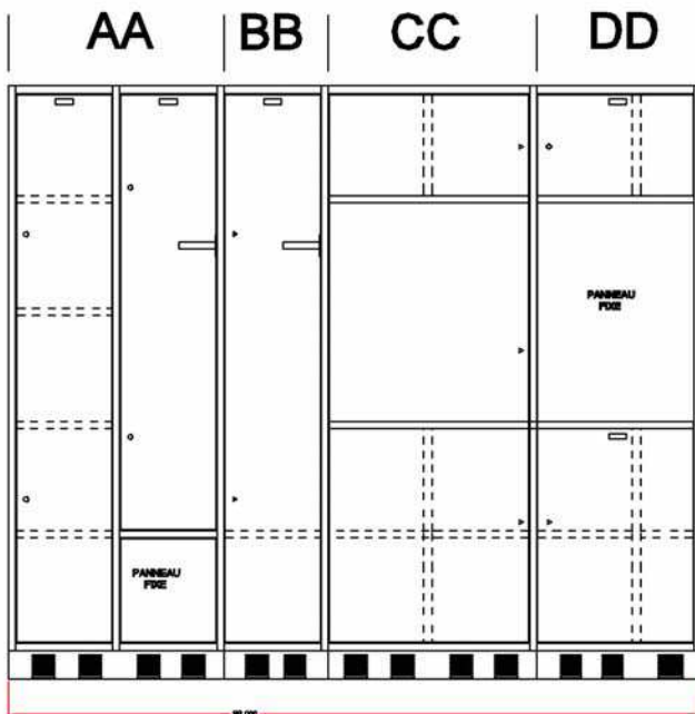
ÉLÉVATION VUE ARRIÈRE/REAR VIEW
