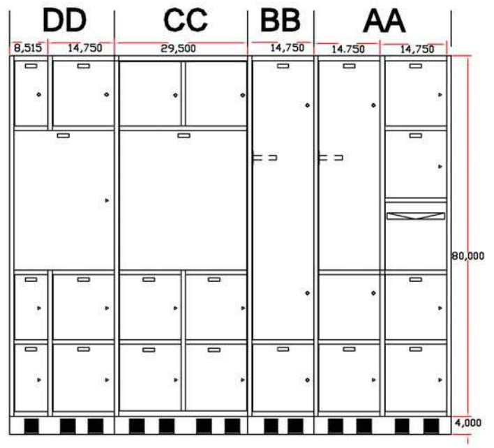
ÉLÉVATION VUE AVANT/FRONT VIEW
